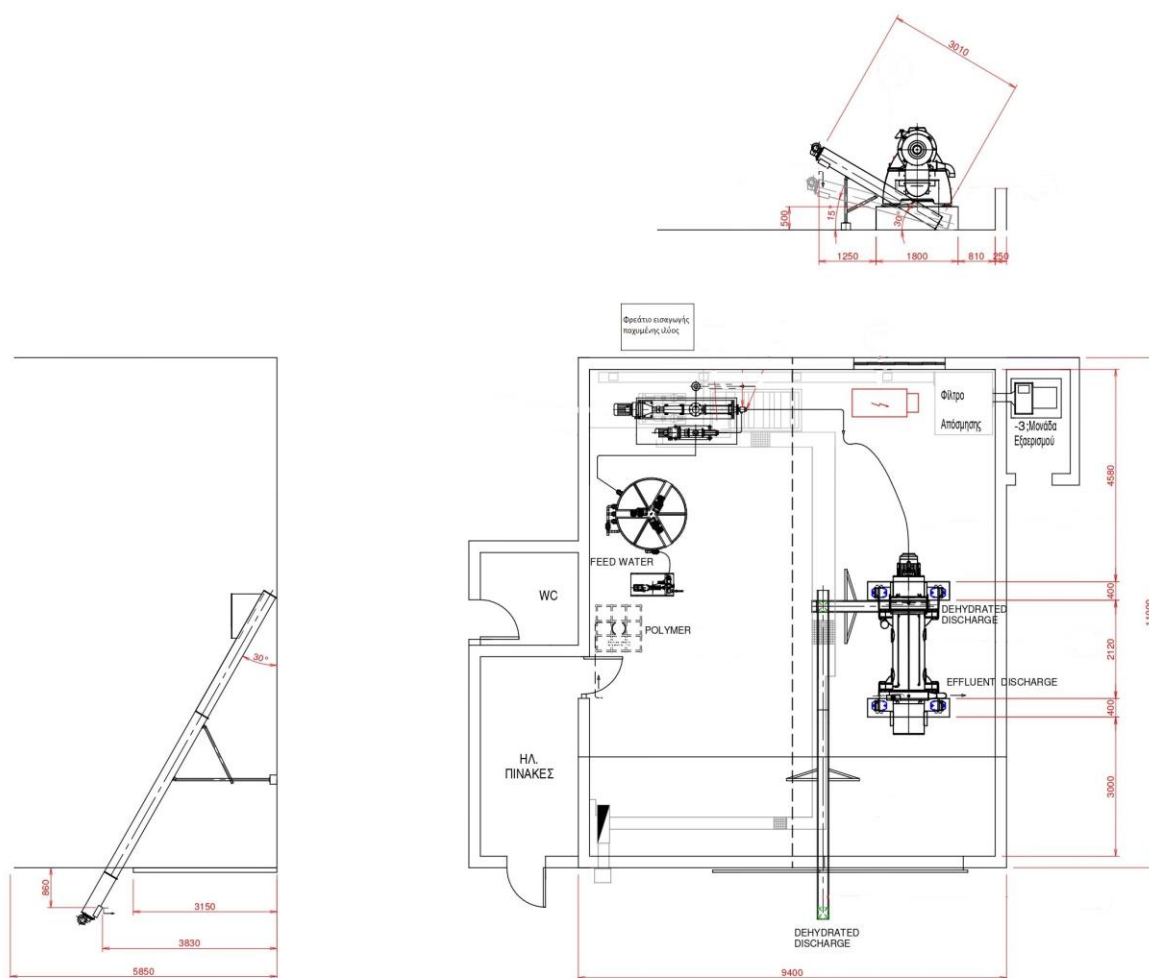
Σχέδιο 1: Ενδεικτική διάταξη του φυγόκεντρικού διαχωριστή και του συνόλου του εξοπλισμού, εντός του υφιστάμενου κτιρίου αφυδάτωσης.
